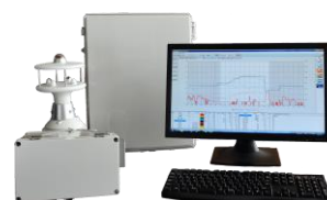
環境制御システム エアロビート (イノチオアグリ株式会社)
